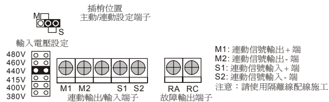
VFDB 4132 設定位置
