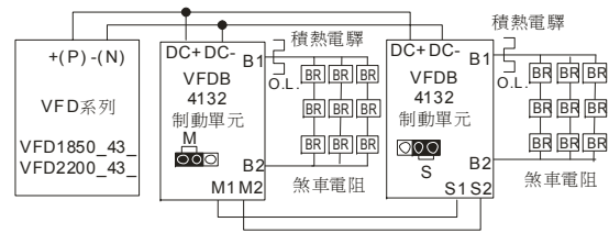
VFD1850_43_使用2台VFDB4132制動單元，每4台使用BR1K5W005 9PCS，每3PCS串聯後再並聯接線
