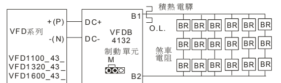
VFD1100_43_使用1K2W008 18PCS，每3PCS串聯後再並聯接線
