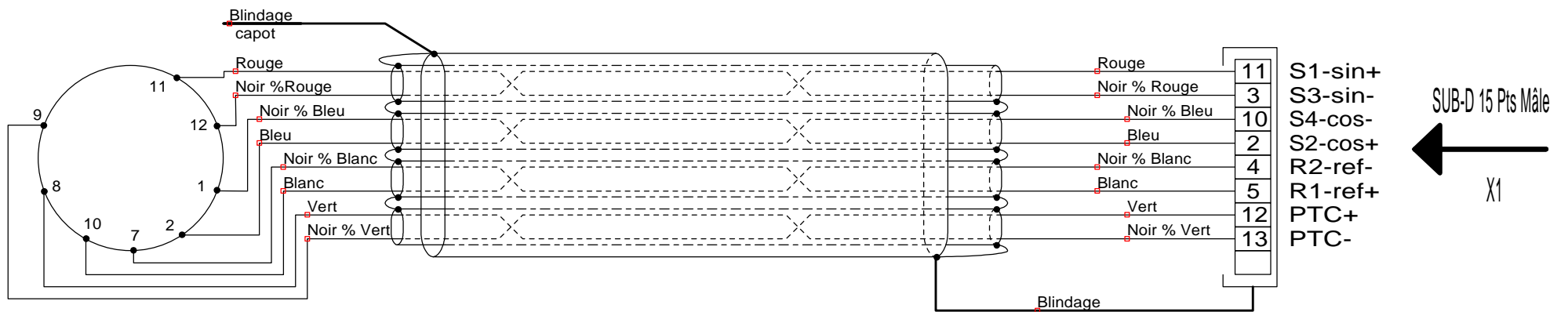
Connecteur M17
