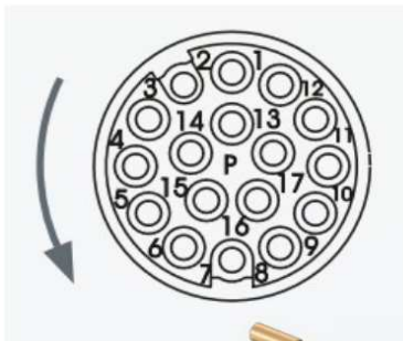
Connecteur M17
