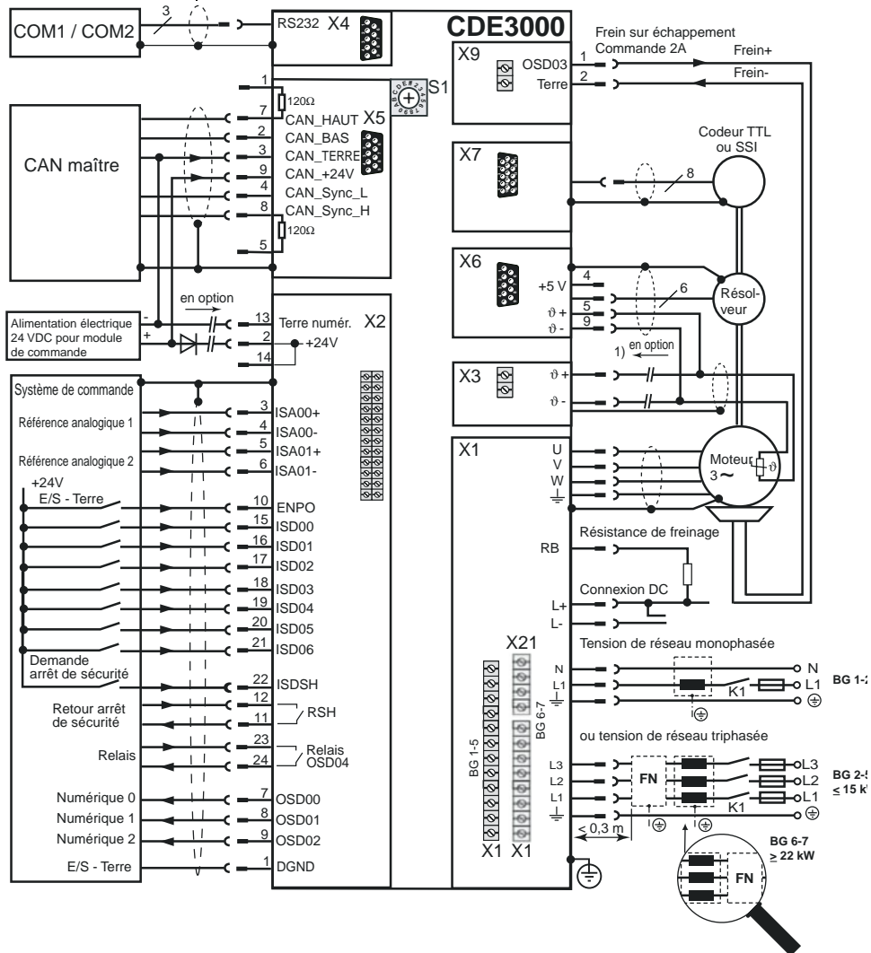
Fig. 3.1 Plan du bornier CDE3000
